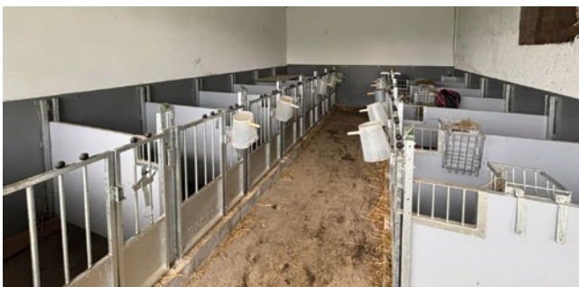
Gruppenhaltung durch gezielte Trennwände
