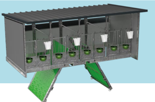
Quattro XXL mit geöffneten EasyClean-Böden
